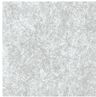
MARL
