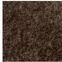
GABBRO
